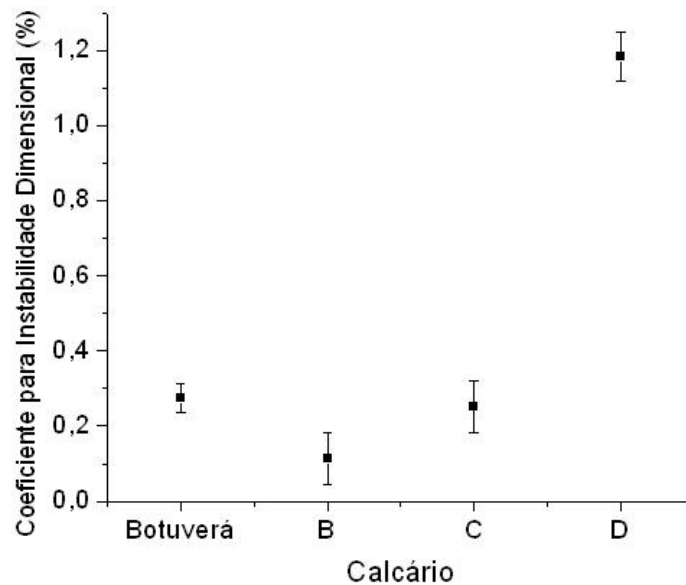
Figura 7 – Contribuição dos calcários para aumento da instabilidade dimensional.
