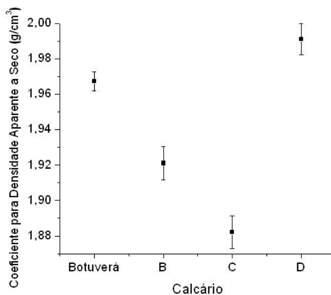
Figura 4 – Contribuição dos calcários para o aumento da densidade aparente a seco da massa.
