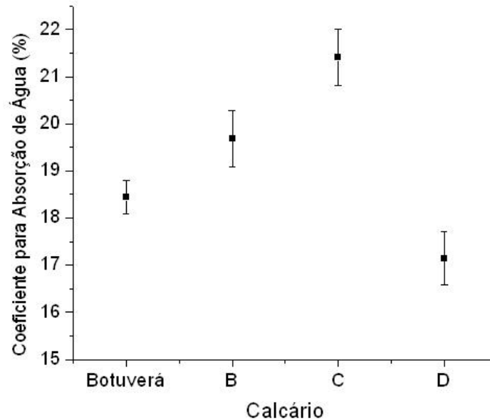
Figura 5 – Contribuição dos calcários para a absorção de água da massa.
