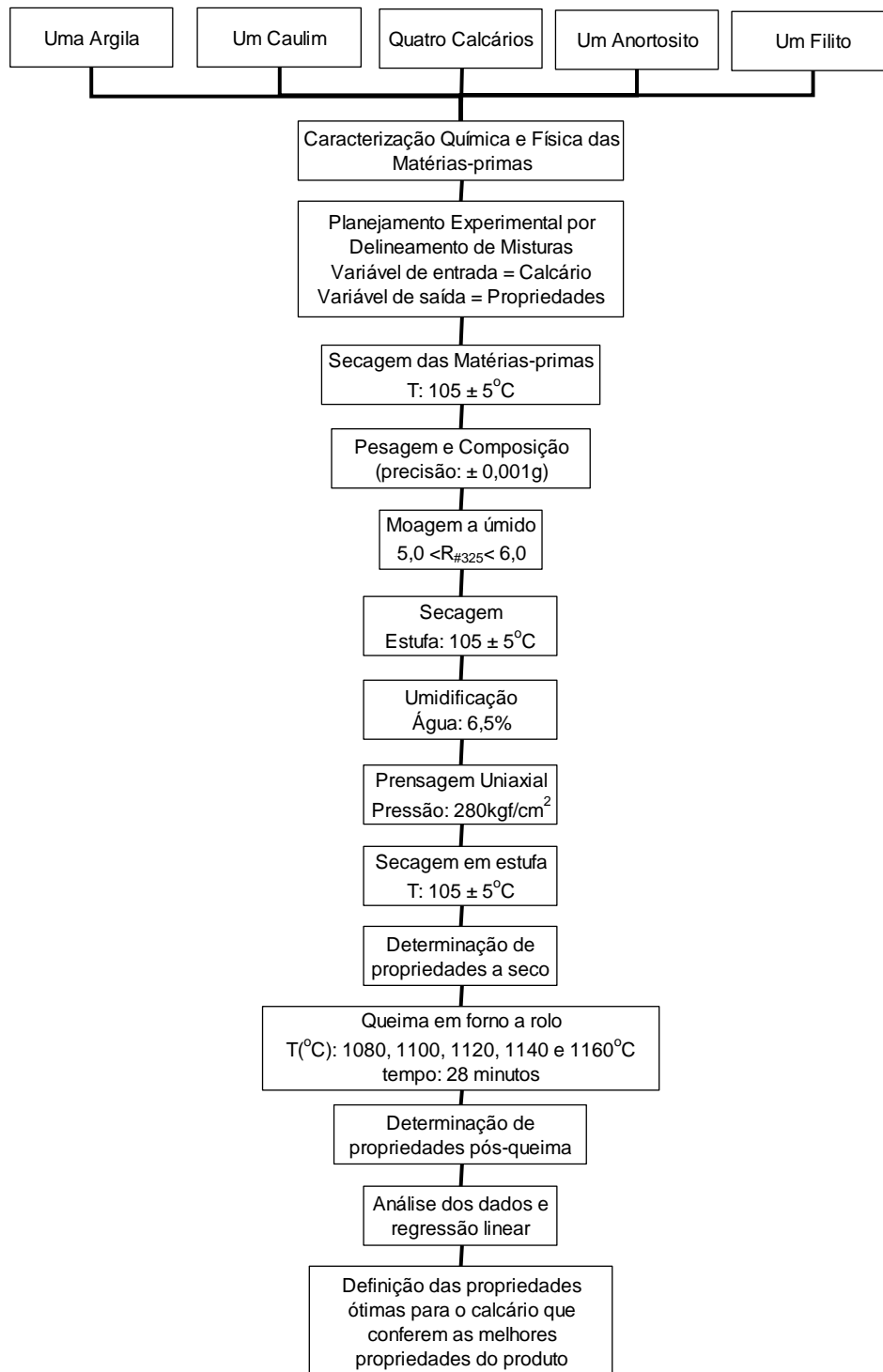
Figura 3 – Fluxograma de processamento do experimento guiado pelo delineamento de misturas.
