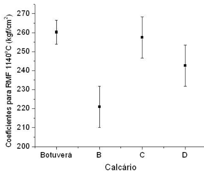
Figura 6 – Contribuição dos calcários para a resistência mecânica a flexão da massa queimada à 1140°C.
