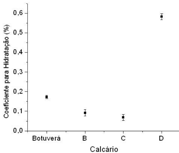
Figura 8 – Contribuição dos calcários para o aumento da hidratação de fases amorfas e/ou vítreas.
